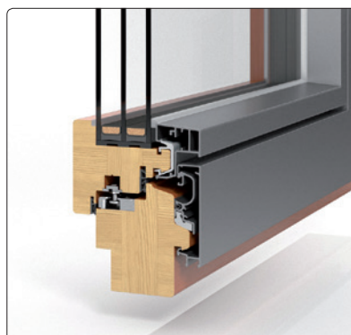
PaXoptima 78 mit flächen- bündigem Profil (links), Flügel kantig profiliert (rechts)
