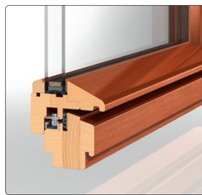
PaXretro 78 mit einer einbruchhemmenden Verglasung (links) und PaXretro 58 (unten)
