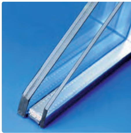
Glasaufbau P4A-Sicherheitsglas
